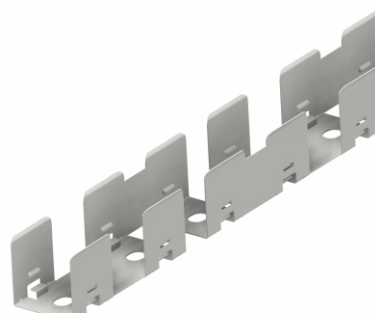
Εύκαμπτο προφίλ INOX για NEON 10x10 INOX bendable Profile for NEON 10x10
