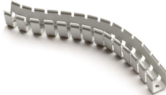
Εύκαμπτο προφίλ INOX για NEON 8x15 INOX bendable Profile for NEON 8x15
