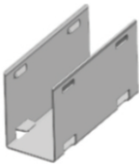
Στήριγμα INOX για NEON 8x15 INOX clip for NEON 8x15
